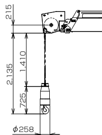
3段フルオートジブ
